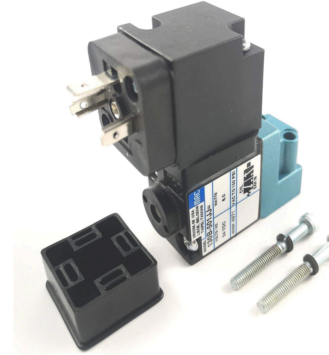
Universal pilot valf 24V/DC/NO/NC
